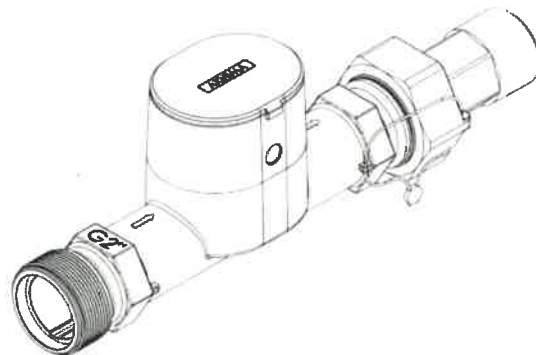
Fig. 2c) Sealing DN40
